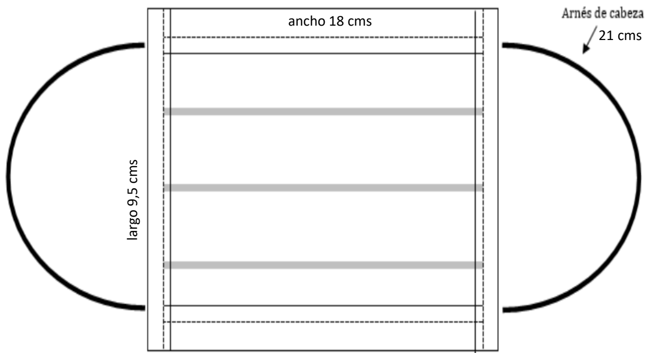
Figura 1 - Ejemplo de mascarilla higiénica terminada con arnés de material elástico con sujeción en las orejas
